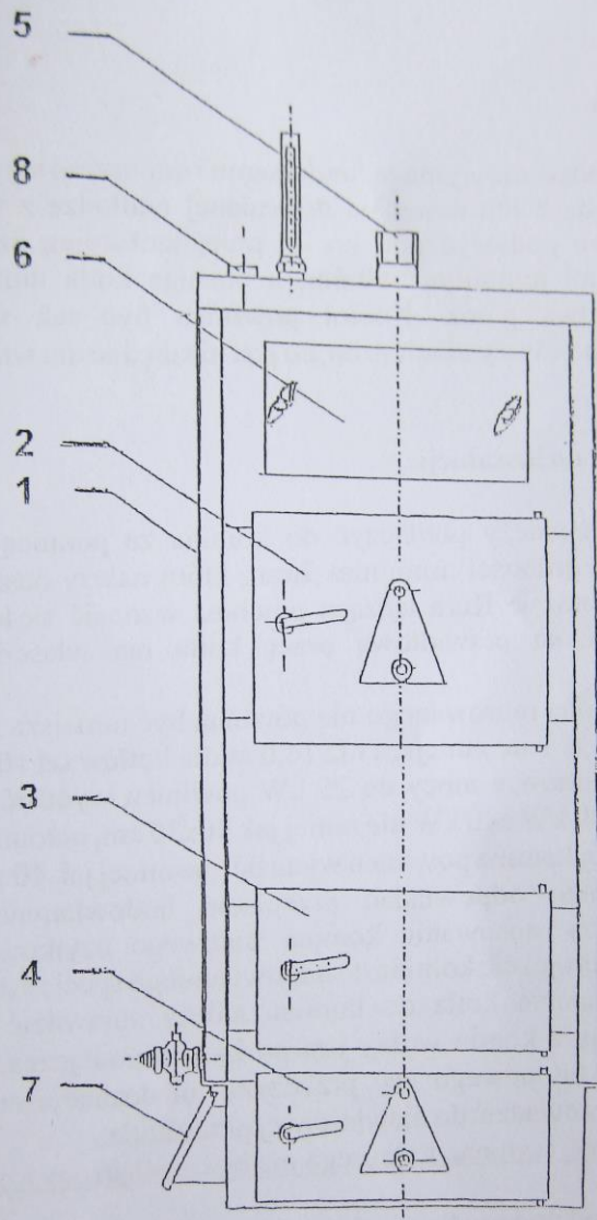
Rys. 2 Schemat konstrukcyjny kotła „KOTEK - SLUPEK”
